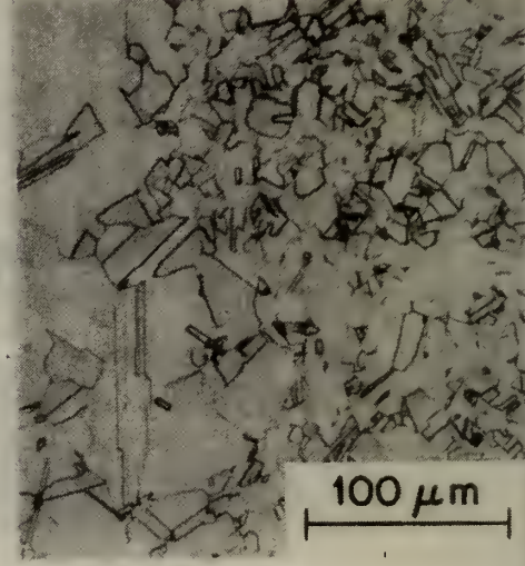
Incoloy 800, 250 X
